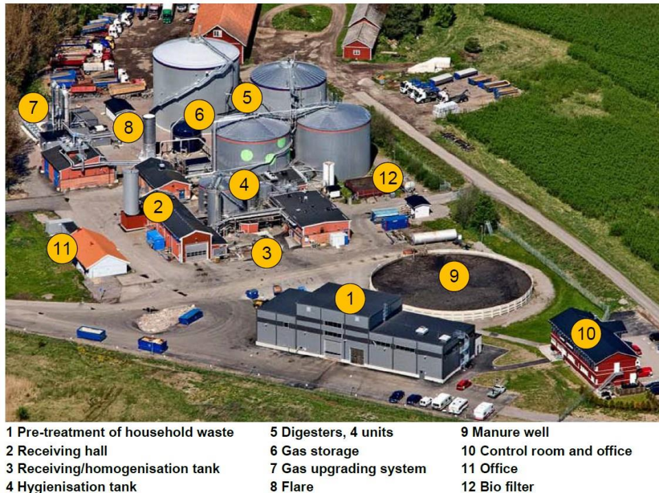
Figure 10. Layout of Åby biogas plant, Tekniska Verken i Linköping.
