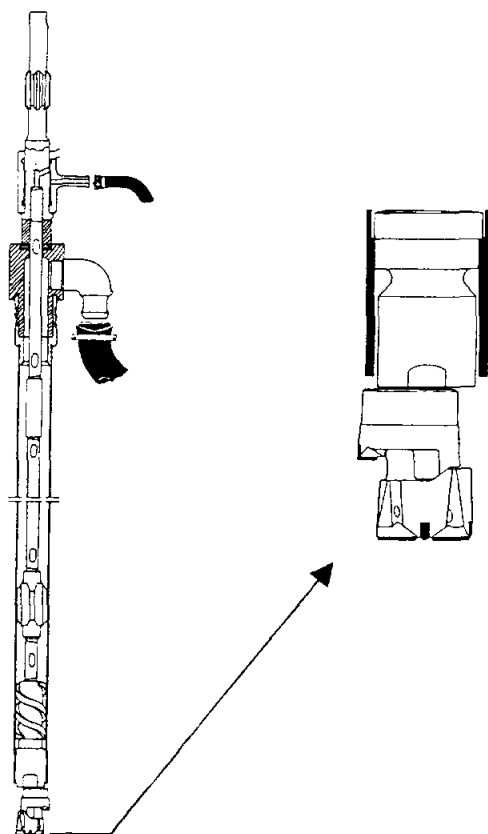
Figur 5.1. ODEX-utrustning (Atlas Copco 3'' ODEX).
