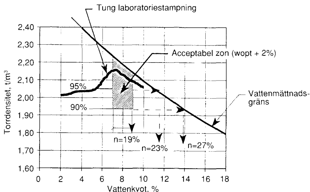
Figur 4.1. Tillåtna variationer i tätjordens torrdensitet i samband med byggandet.
