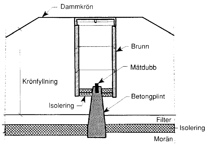
Figur 3.4. Mätdubb i tåtkärnans krön.
