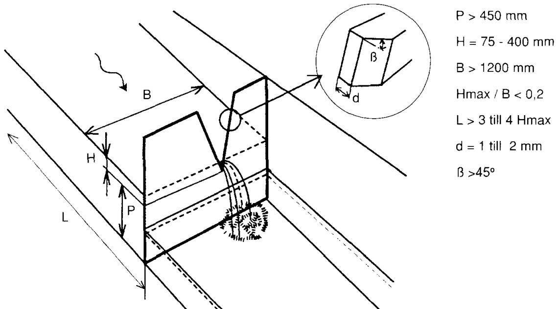
Figur 3.1. Triangulärt mätöverfall i kanal.
