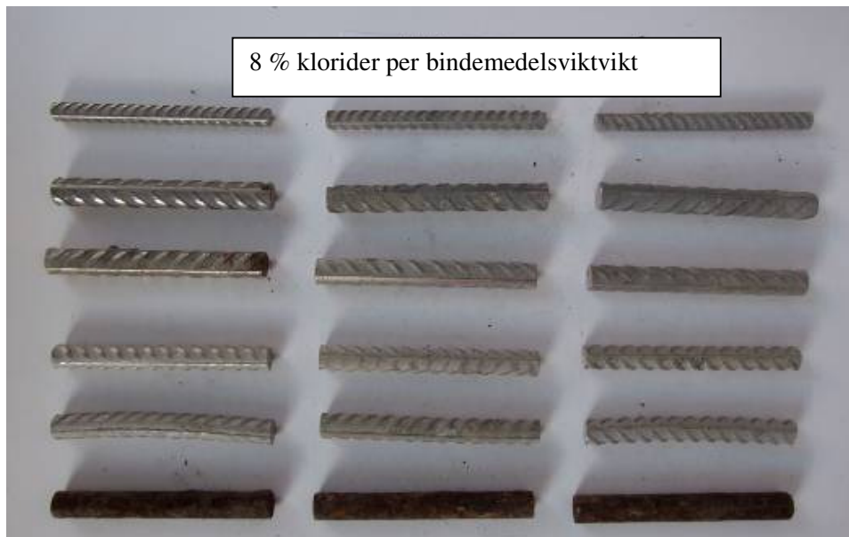
Figur 33 Utseendet hos provstänger av rostfritt stål och kolstål efter två års exponering utomhus ingjutna i betong (PFA C32/40, vbt 0,45) med 8 % klorider
