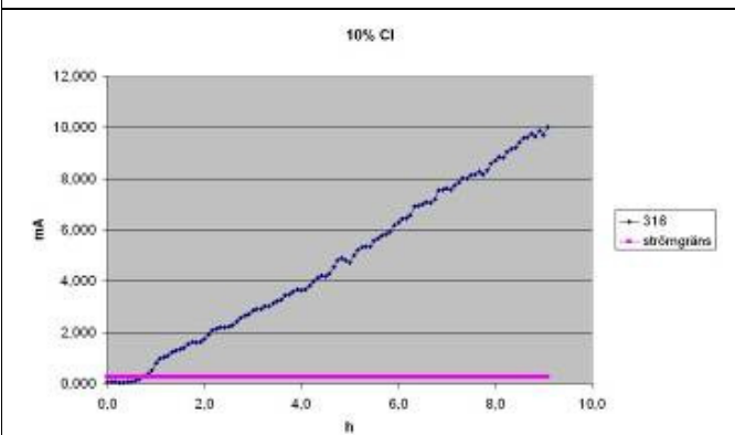
c) 316 (EN 1.4436)
