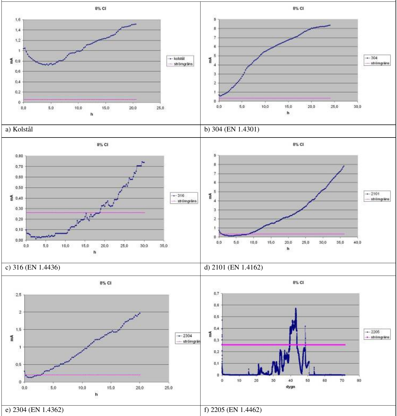
Figur 45 8 vikt-% Cl per cementvikt
