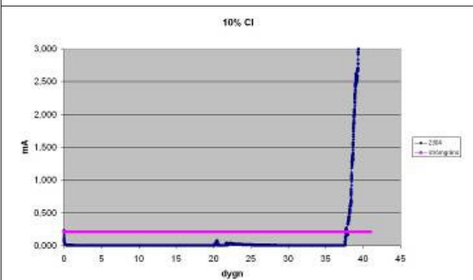
e) 2304 (EN 1.4362)
