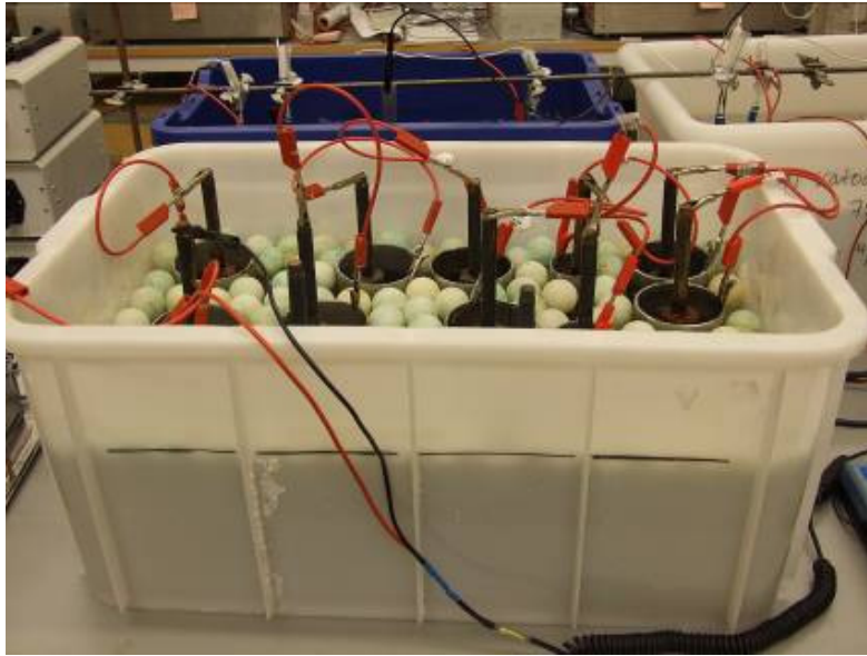
Figur 14 Försöksuppläggning på laboratorium
