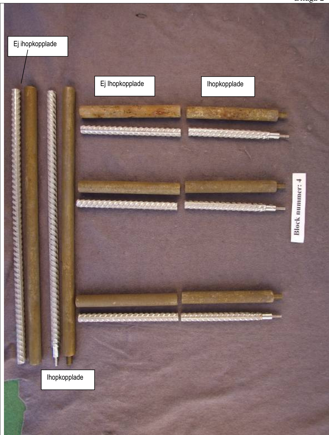
Betongblock 4: PFA C32/40 (CEMIIB-V) Rostfri stålqualität: EN 1.4362 Täckande betongskikt: 15 mm Kloridhalt: 3 % per bindemedelsvikt Exponeringstid: 2 år
