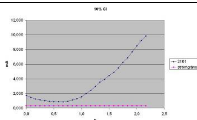
d) 2101 (EN 1.4162)
