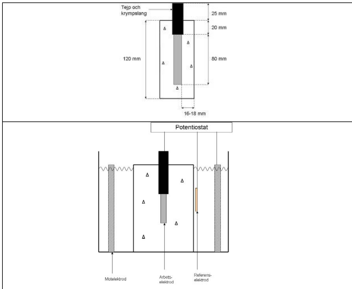
Figur 16 Schematisk beskrivning av försöksuppställning
