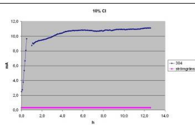
b) 304 (EN 1.4301)
