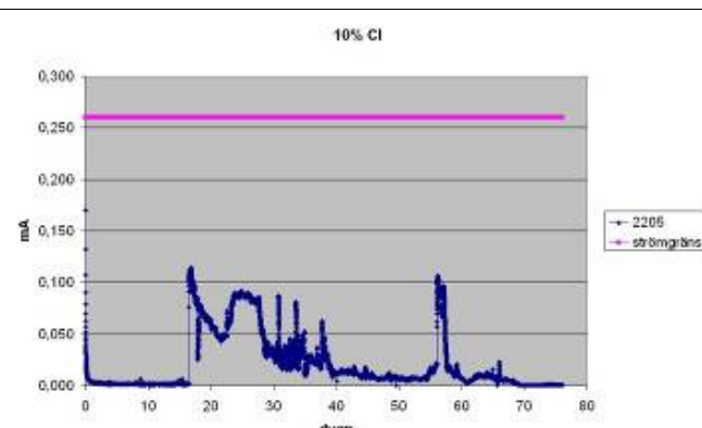
f) 2205 (EN 1.4462)
