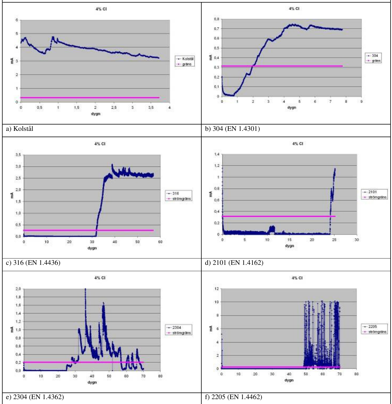
Figur 47 4 vikt-% Cl per cementvikt
