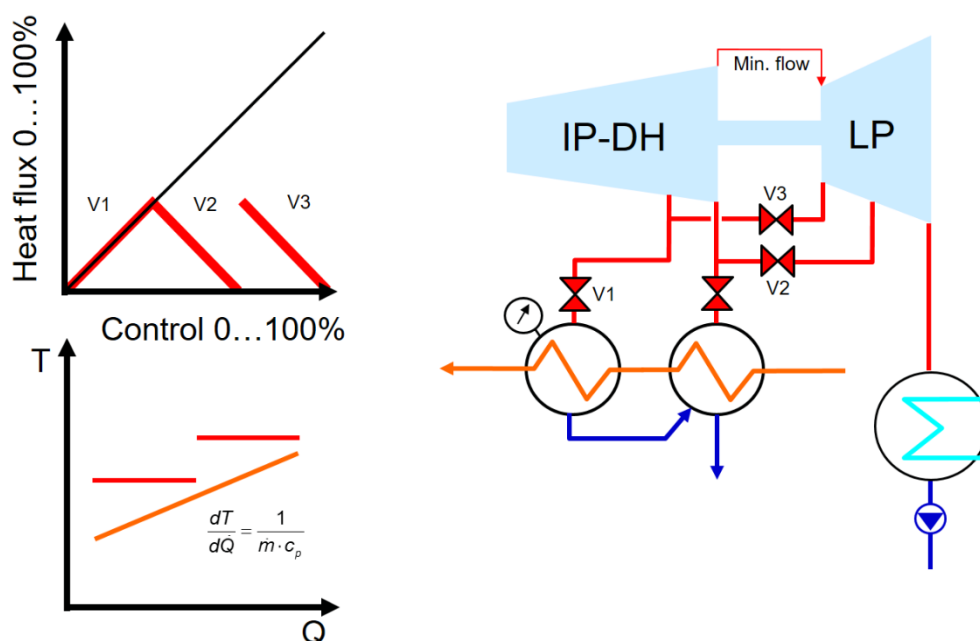
Figur 8-2. Kondenssvanskoppling
