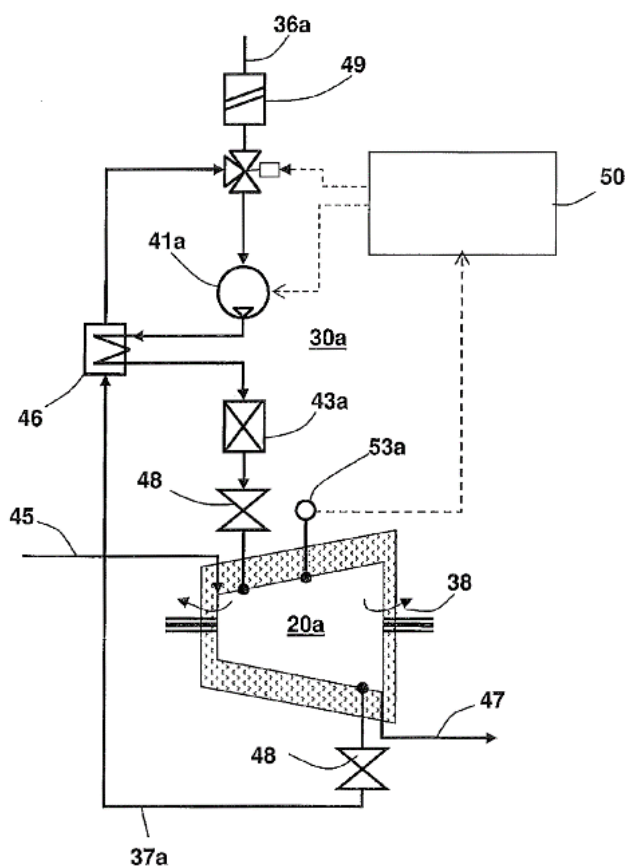
Figur 8-11. Koppling hetluftsvärmning (från GE/Alstom patent)
