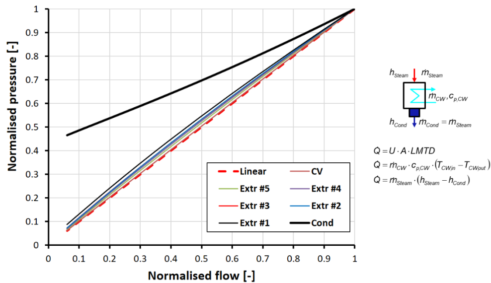
Figur 8-9. Trycknivåer
