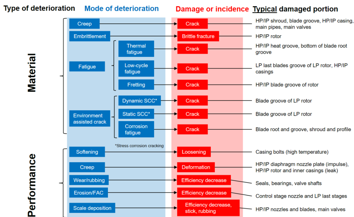
Figur 10-1. Typiska skador
