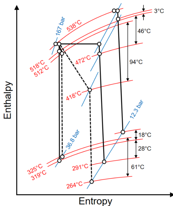
Figur 8-6. Expansionsförlopp för olika reglerformer
