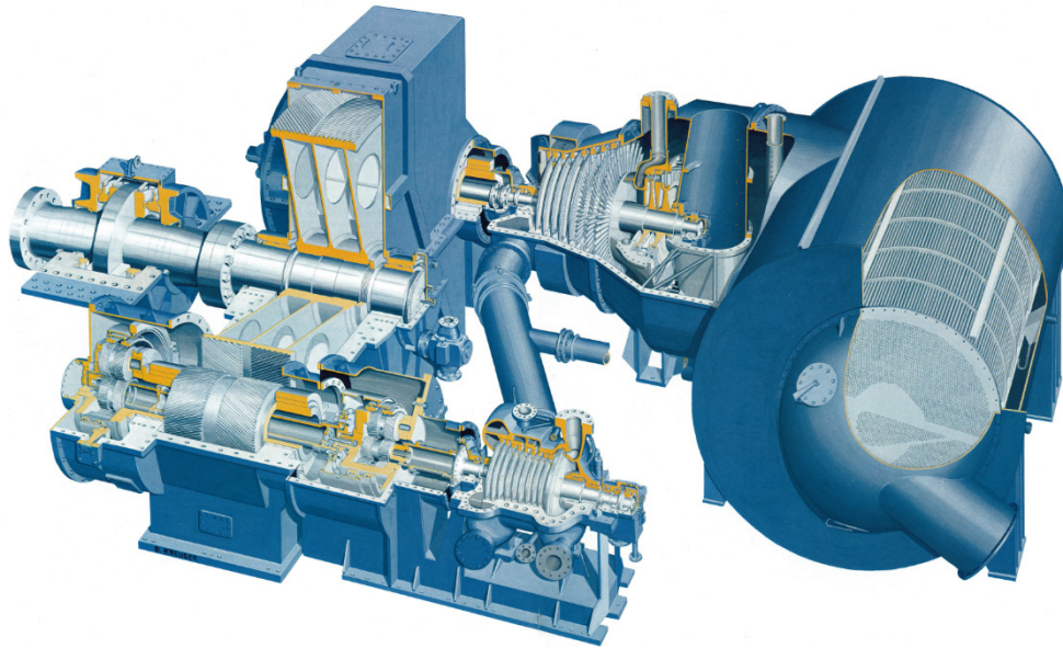
Figur 1-3. Stal-Laval AP-turbin för fartygsdrift
