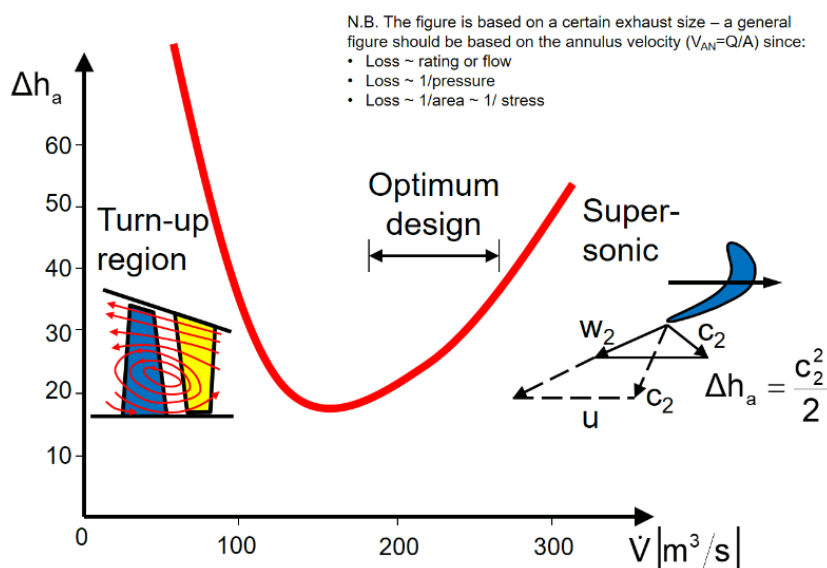
Figur 8-7. Typisk avloppsförlustkurva
