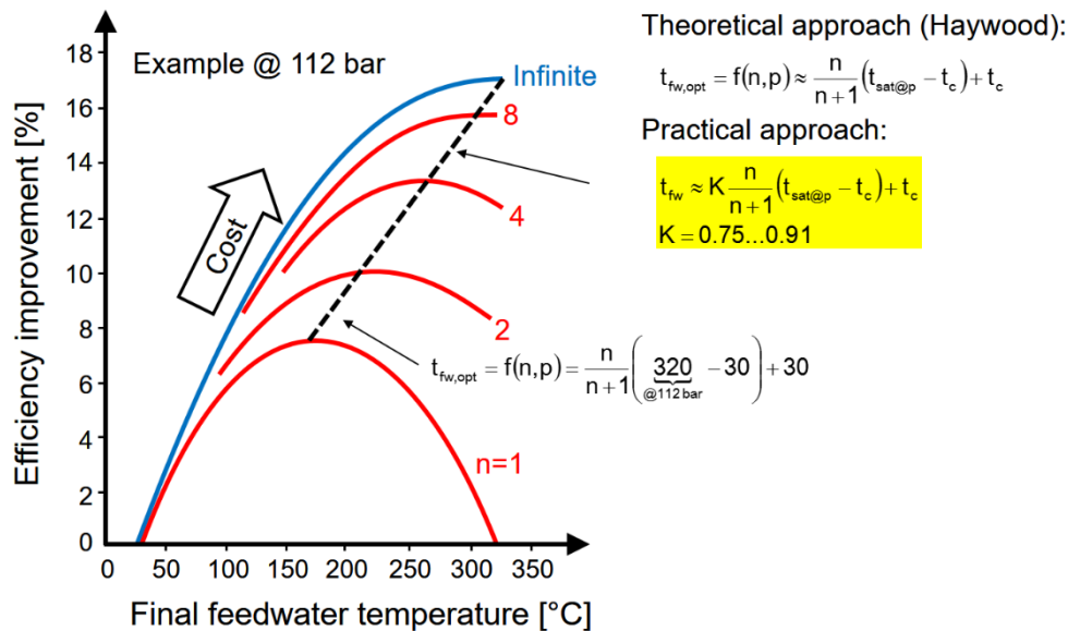
Figur 5-4. Exempel på vinst med matarvattenförvärmning vid 112 bar a ångtryck.
