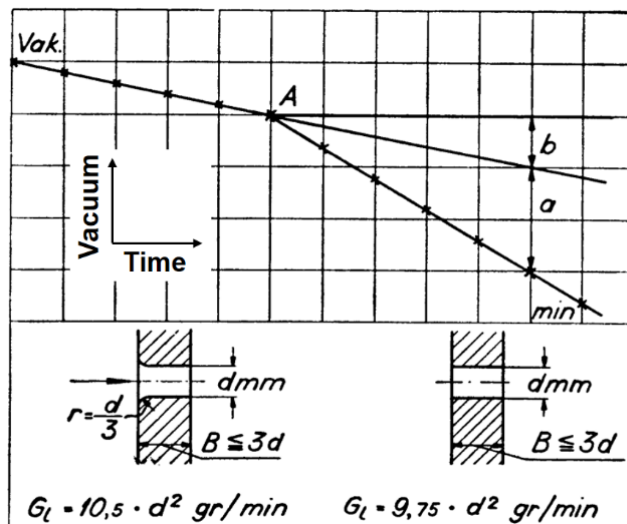
Figur 12-2. Vacuumfallsprov
