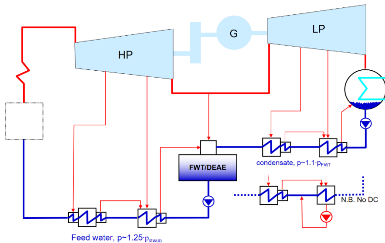
Figur 8-8. Exempelcykel
