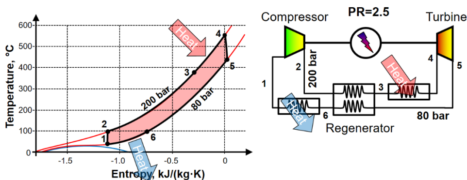
Figur 8-2 Superkritisk CO 2 -process
