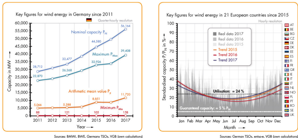
Figur 1-3 Vindkraftsstatistik Tyskland 2016-2017 samt vindkraftsproduktion i 21 EU-länder 2015-2017 (VGB)
