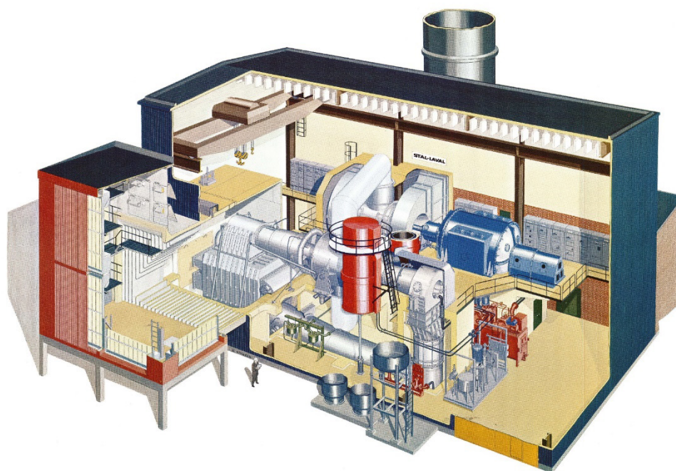
Figur 2-1 STAL-LAVAL GT120 (STAL-LAVAL) – exempelvis Stallbacka, Kimstad, Värtna och Halmstad
