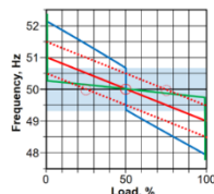
Figur 1-1 Frekvensreglering elnät – Baseras på diverse källor (tex SVK)
