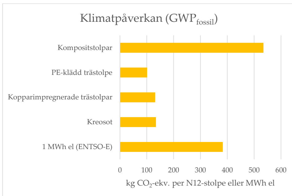
Figur 15 - Jämförelse av ledningsstolpars totala klimatpåverkan över sin livscykel med produktion av 1 MWh europeisk el.
