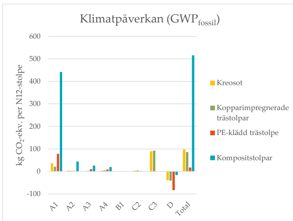
Figur 12 - Klimatpåverkan för stolpmaterialen med hänsyn taget till återvinningspotentialen för respektive stolpe (modul D enligt EN15804).
