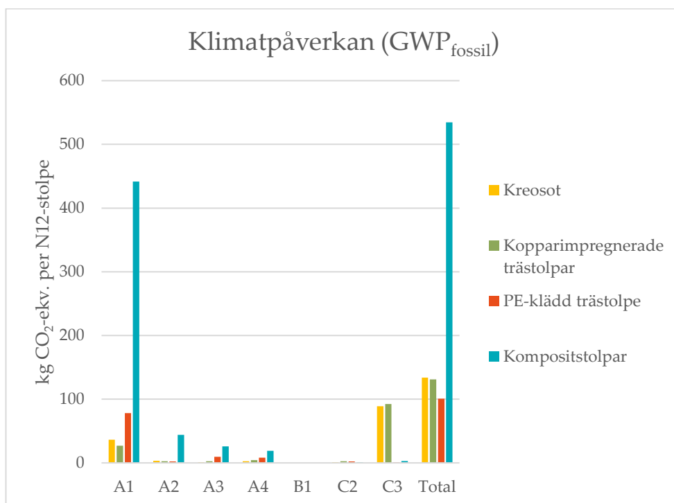
Figur 4 - Klimatpåverkan för respektive stolpmaterial uttryckt i kg CO 2 -ekv per stolpe.
