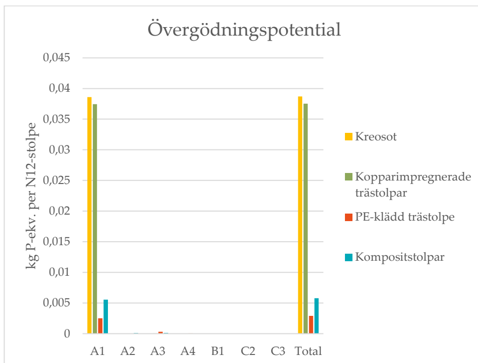
Figur 6 - Övergödningspotential för respektive stolpmaterial uttryckt i kg P-ekv per stolptyp.
