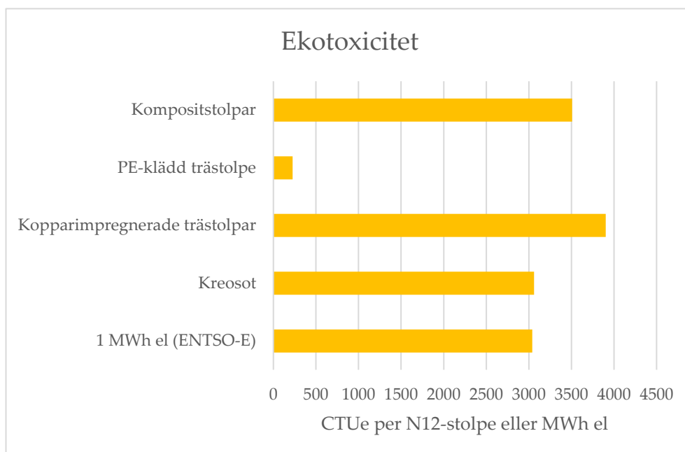
Figur 17 - Jämförelse av ledningsstolpars ekotoxicitetspotential med produktion av 1 MWh europeisk el.
