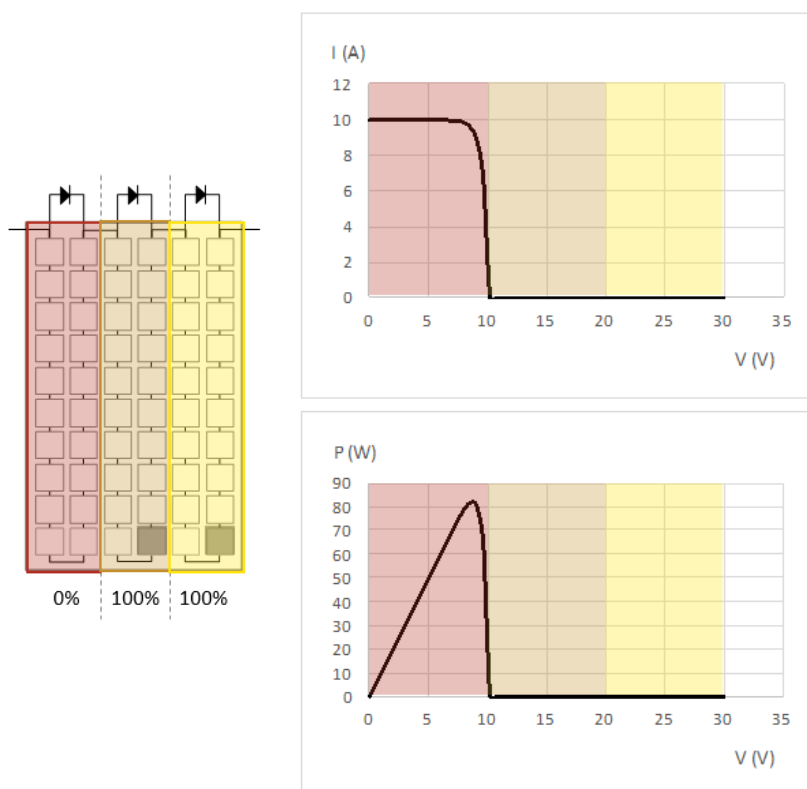
Figur 42 Två slingor är helt skuggade.
