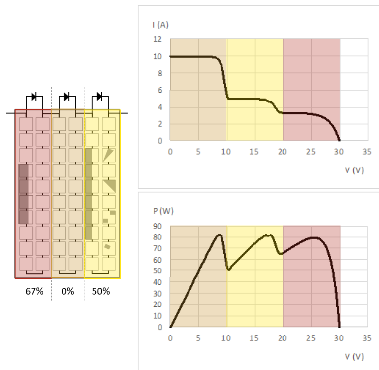
Figur 39 Heterogen skuggning av modul, 67 %, 0 % och 50 %.
