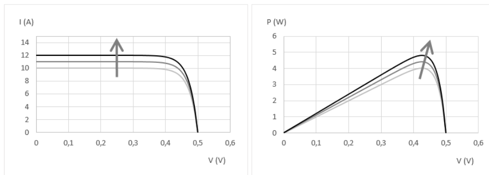
Figur 21 IV-kurvans och PV-kurvans beroende av solinstrålningen.
