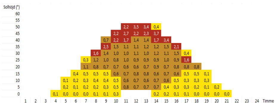
Figur 62 Procentandel av global solinstrålning mot en yta som lutar 40° mot söder under medelår i Stockholm.
