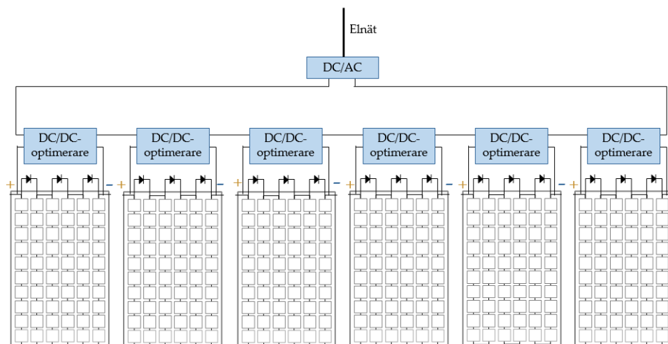
Figur 29 Sträng med moduloptimerare.
