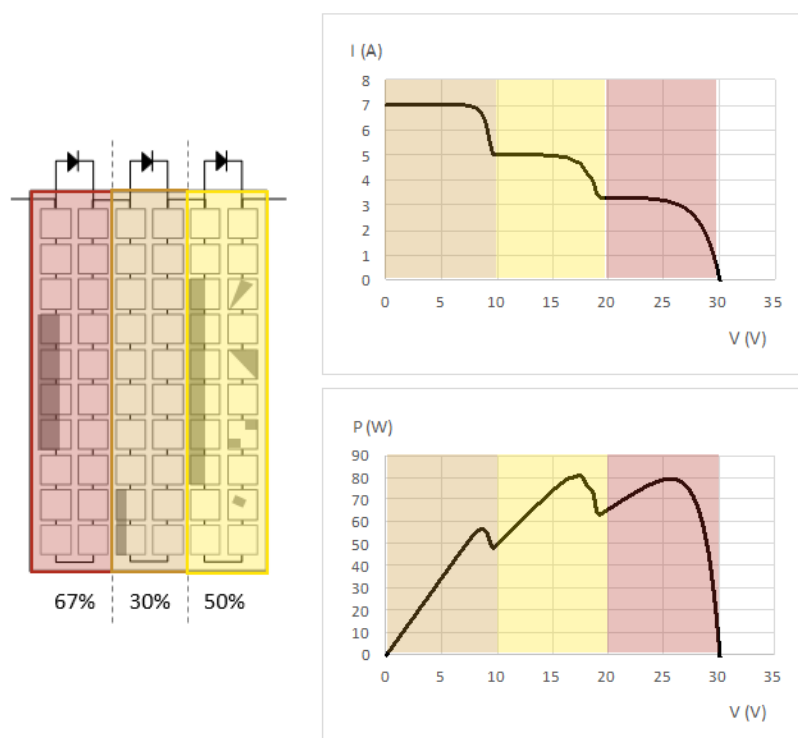
Figur 41 Heterogen skuggning av modul, 67 %, 30 % och 50 %.
