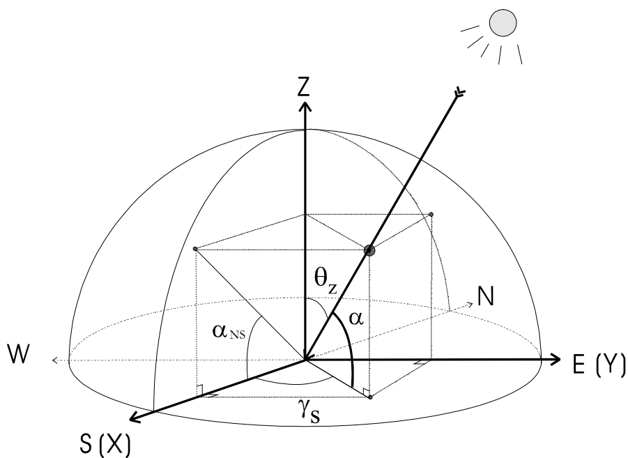
Figur 10 Vinkeln \alpha är solhöjden, \gamma_s är solens asimetvinkel och \alpha_{NS} är den effektiva solhöjden.
