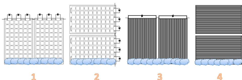
Figur 33 Vertikal respektive horisontell orientering vid snö på kristallina kiselmoduler och tunnfilmmoduler.
