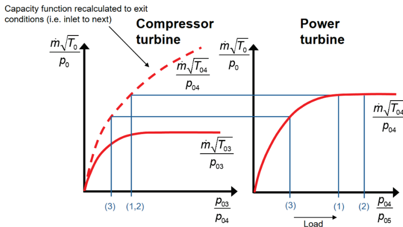
Figur 4-3 Matching kompressor- och kraftturbין [9]
