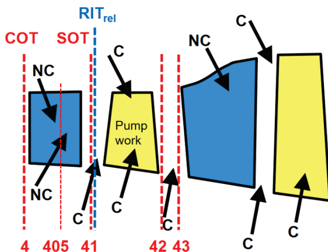
Figur 4-5 Definitioner av eldningsstemperatur(er) [9]
