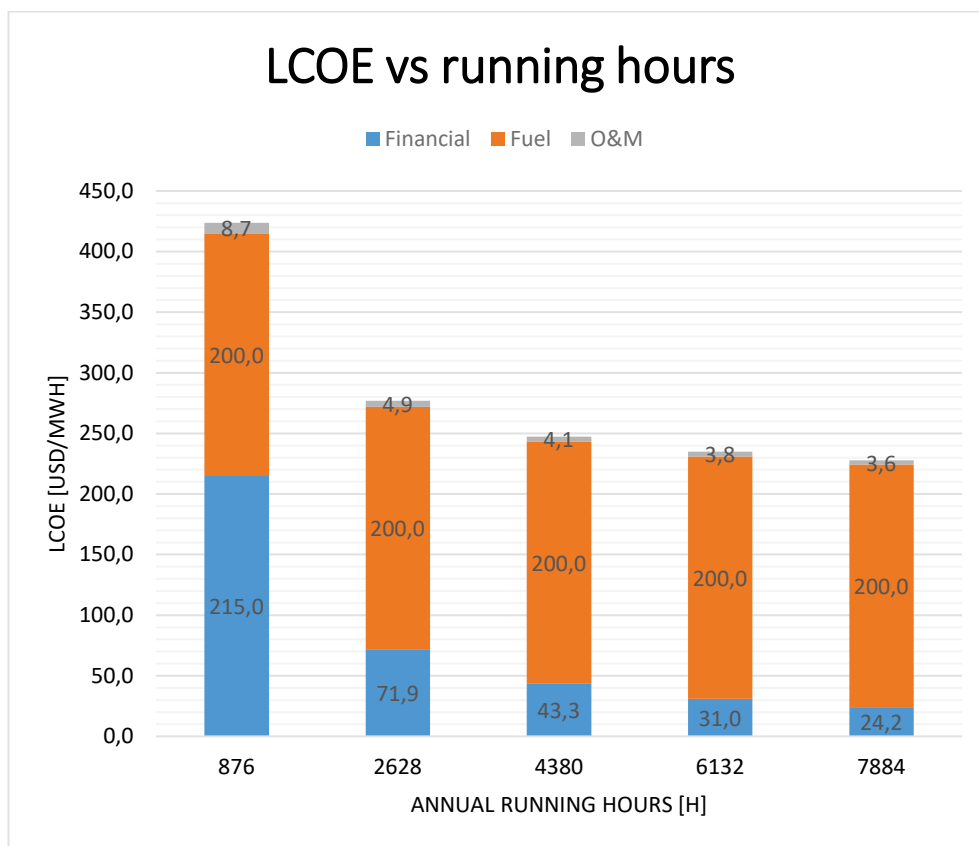
Figur 10-6 LCOE s.f.a drifttid - Vätgas kombicyclel @4 USD/kg
