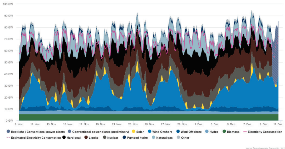
Figur 1-2 Produktionsmix Tyskland december 2017.
