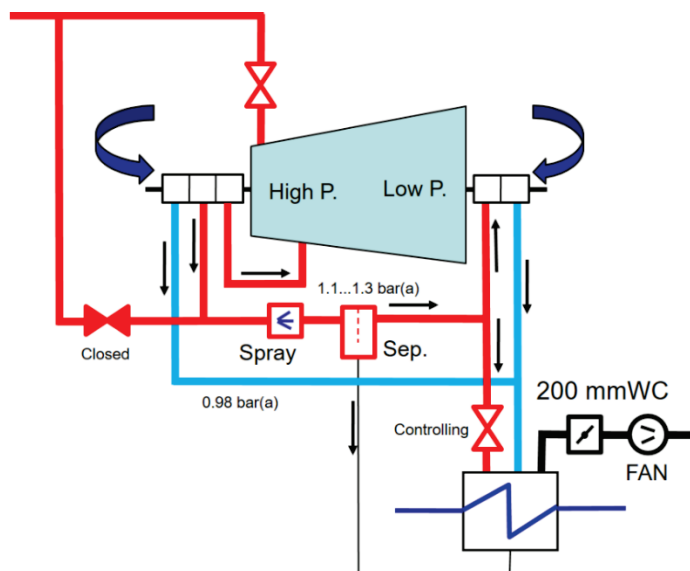
Figur 14-4. Principskiss glandsystem
