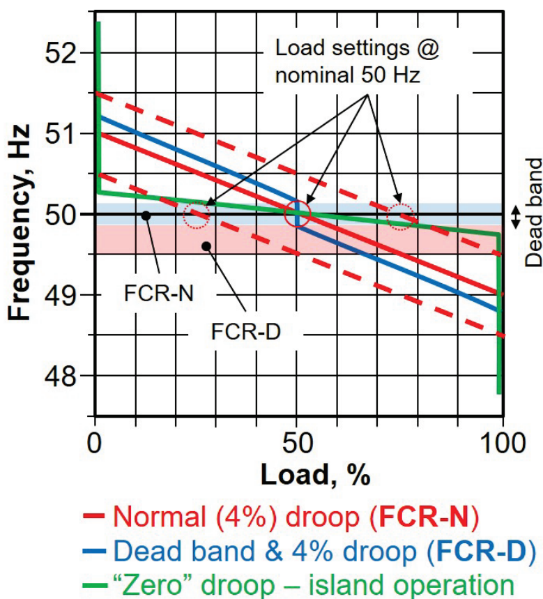
Figur 7-2. Principskiss frekvensreglering
