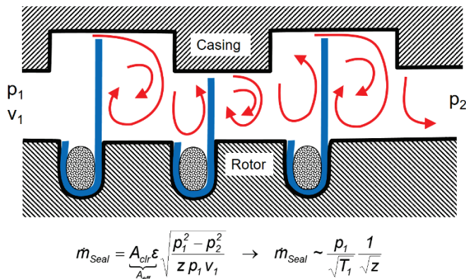
Figur 14-3. Principskiss axeltätning
