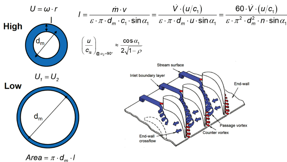
Figur 6-3. Växlad respektive oväxlad turbin
