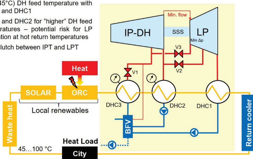
Figur 15-1. Flexibelt 3:e generationens kraftvärmeanläggning
