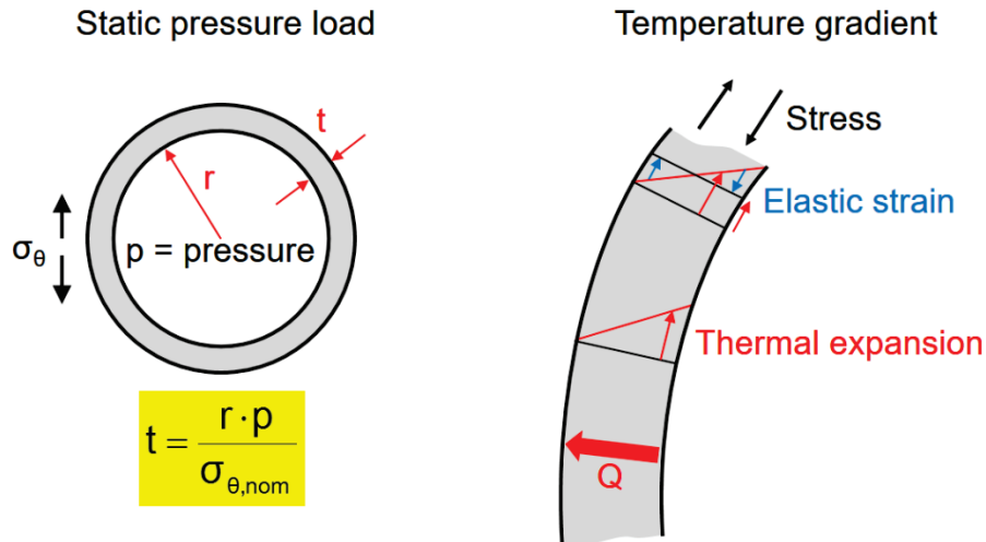
Figur 10-4. Temperaturinducerad tangentialspänning
