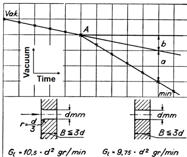
Figur 14-2. Vacuumfallsprov
