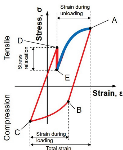
Figur 10-6. Spänning- och töjningsloop
