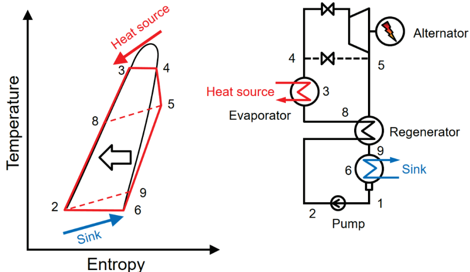
Figur 15-3. Typisk ORC-cykel
