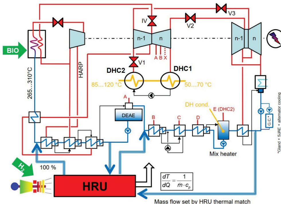
Figur 15-2. Koppling motsvarande Avedöre #2 (AVV2)
