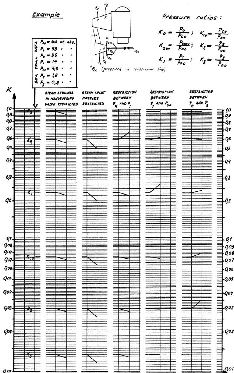
Figur 14-1. Övervakning av trycknivåer i turbinen
