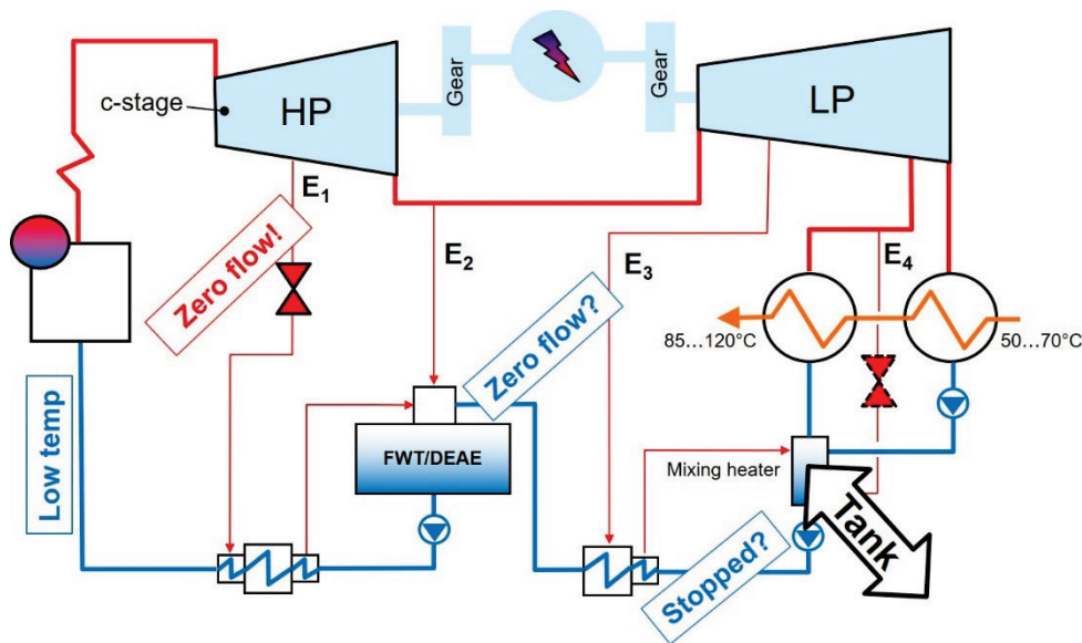
Figur 10-16. Effektökning med förvärmastopp
