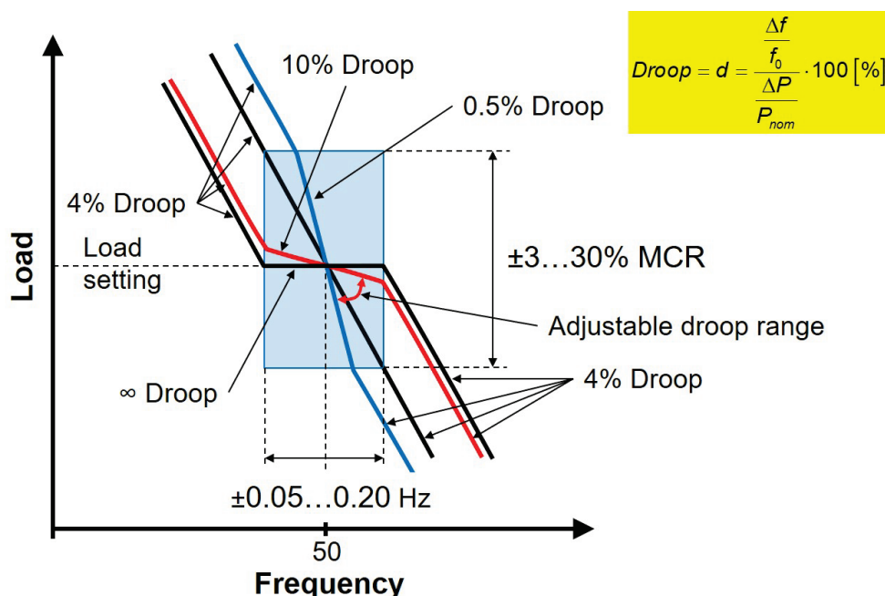
Figur 7-3. Principskiss frekvensreglering med varierande droop (CEGB 22 )
