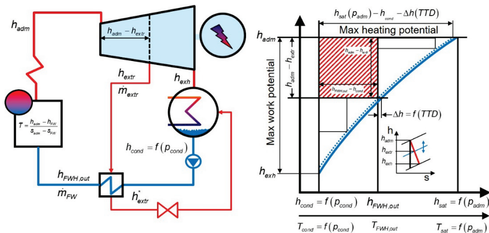
Figur 5-5. Avtappning – val av tryck
