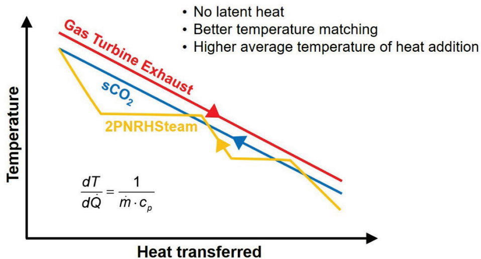
Figur 15-5. T,Q-diagram för vatten och sCO 2
