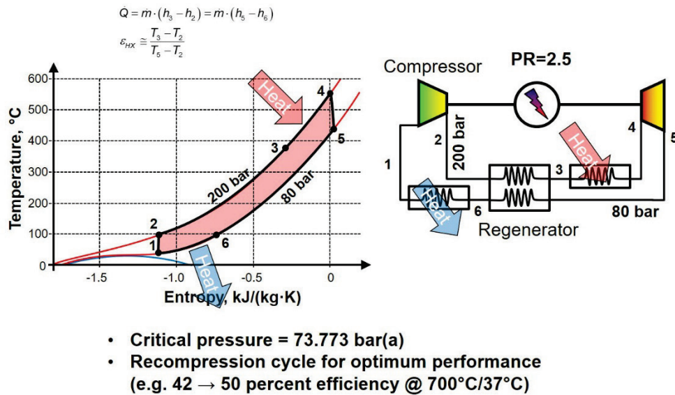
Figur 15-4. Typisk sCO 2 -cykel
