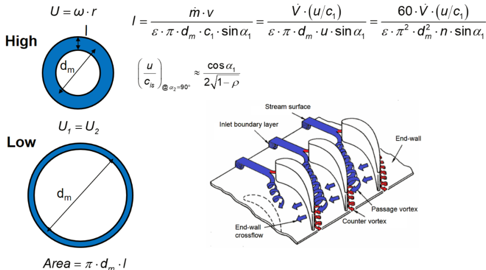
Figur 6-4. Växlad respektive oväxlad turbin
