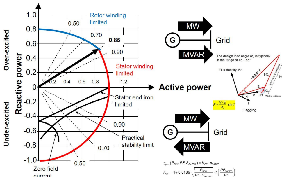
Figur 7-4. Exempel kapabilitesdiagram (P,Q)
