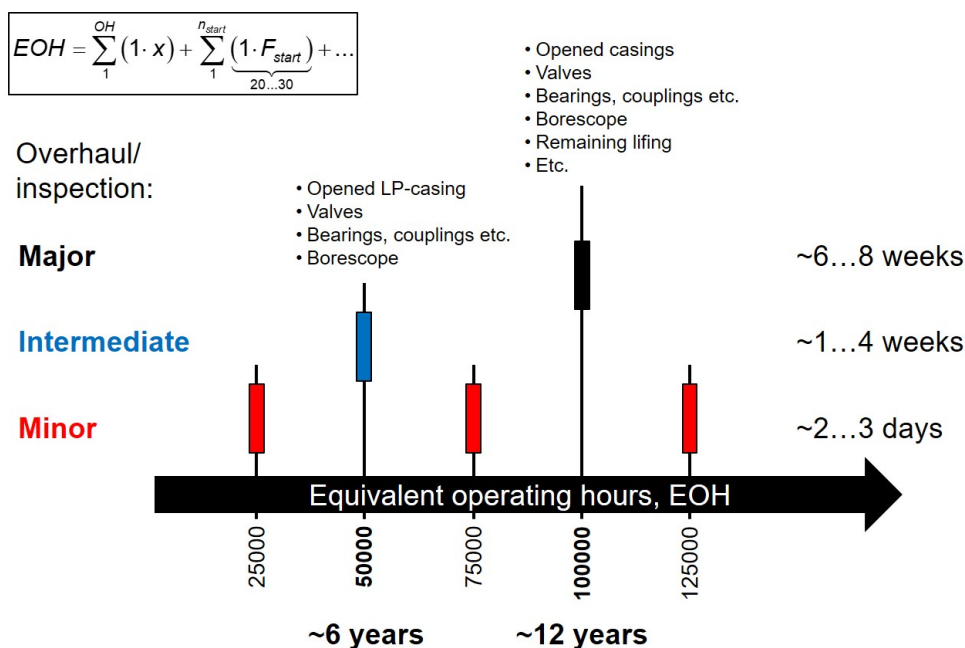
Figur 11-2. Exempel serviceintervall
