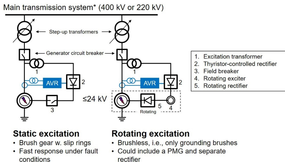
Figur 7-5. Exempel spänningsreglering
