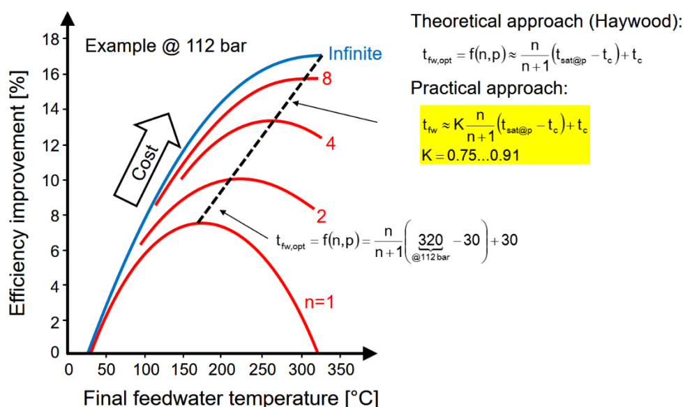
Figur 5-6. Exempel på vinst med matarvattenförvärmning vid 112 bar ångtryck.
