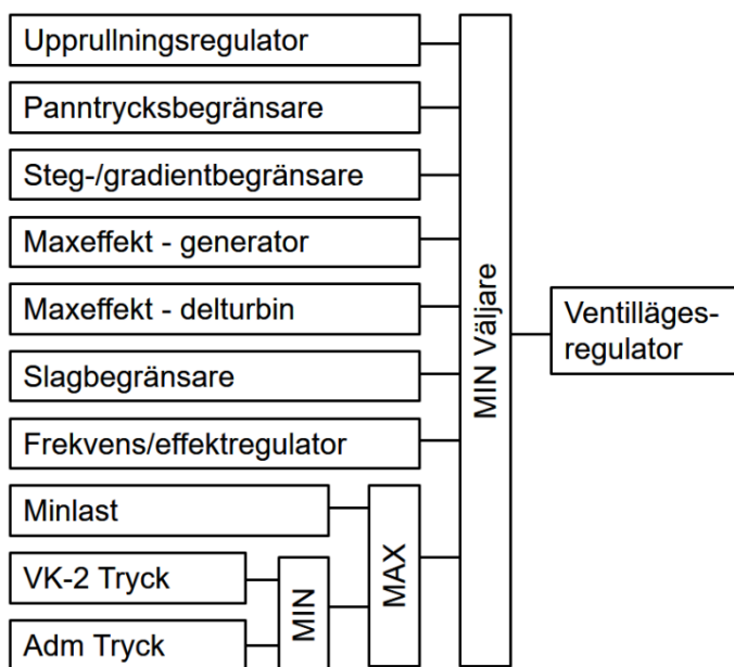
Figur 7-1. Exempel turbinregulator
