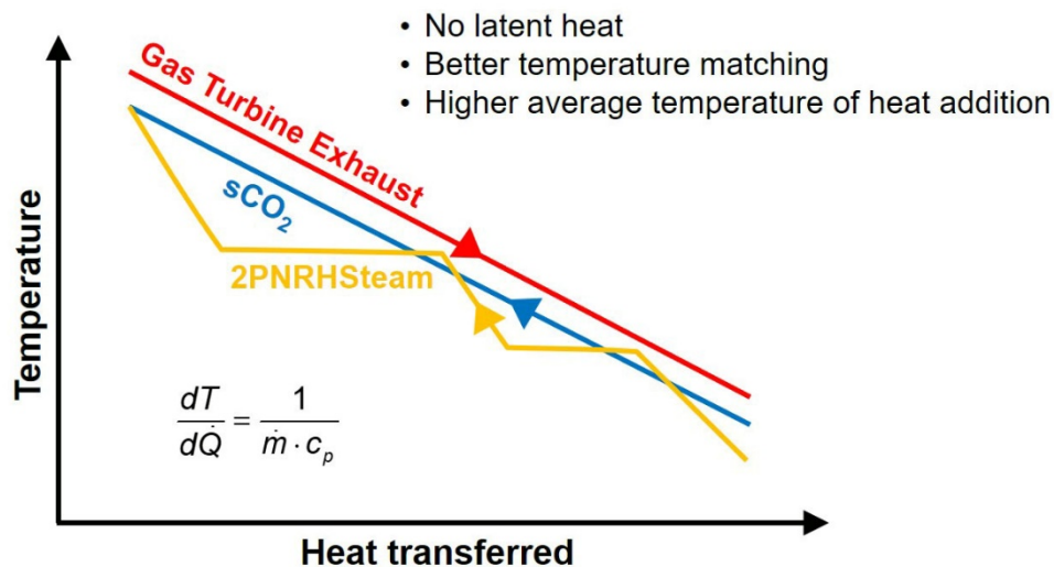
Figur 15-6. T,Q-diagram för vatten och sCO 2
