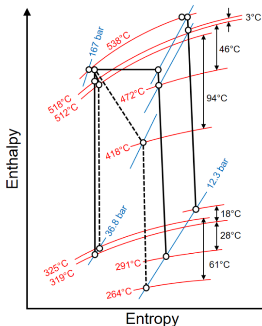
Figur 10-9. Expansionsförlopp för olika reglerformer
