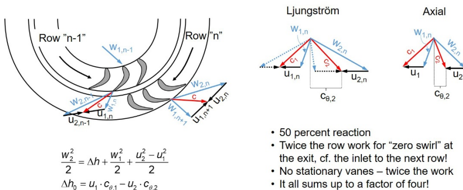
Figur 6-3. Radialturbin - arbetsprincip
