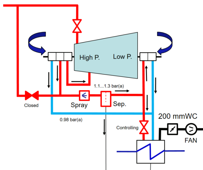
Figur 14-4. Principskiss glandsystem
