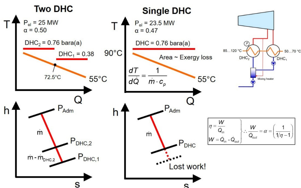
Figur 5-4. Prestanda med en- respektive två värmekondensatorer
