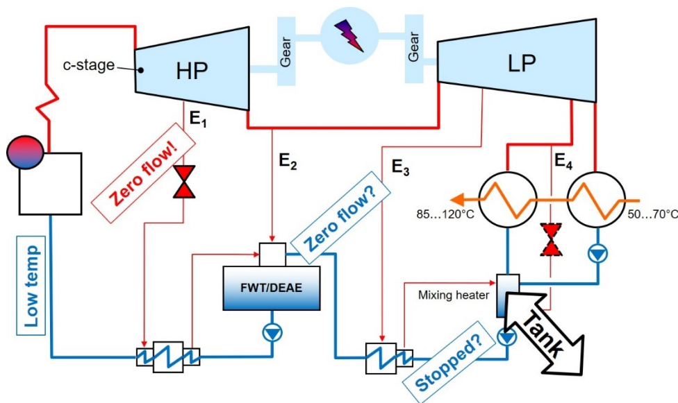
Figur 10-16. Effektökning med förvärmarstopp
