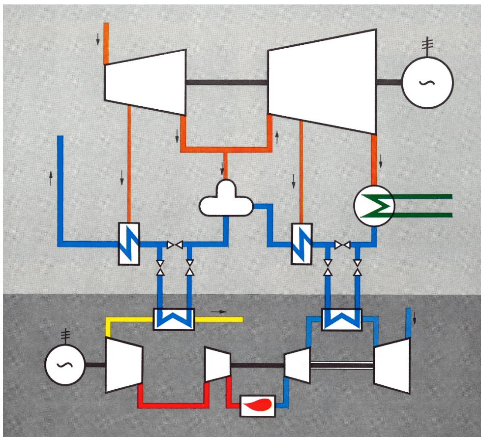
Figur 10-17. Förvärmningskoppling med mellankylad gasturbin (STAL-LAVAL)
