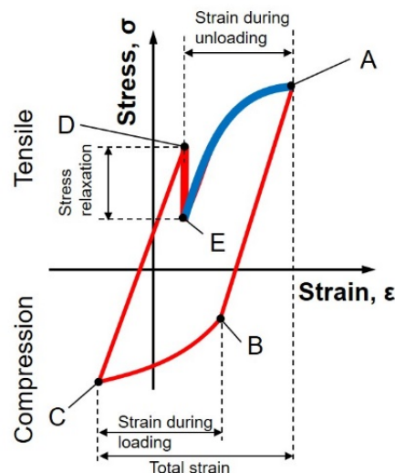
Figur 10-6. Spänning- och töjningloop
