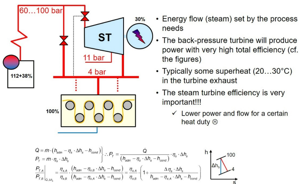
Figur 15-1. Mottrycksanläggning
