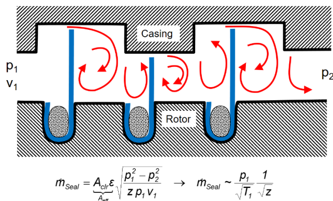
Figur 14-3. Principskiss axeltätning
