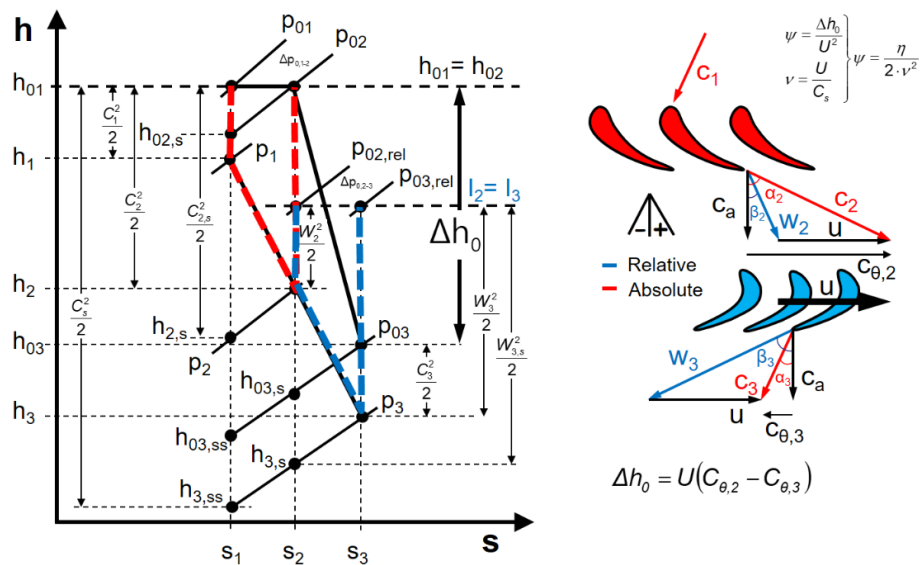
Figur 6-2. Ett turbinsteg i h,s-diagrammet med tillhörande hastighetstriangel
