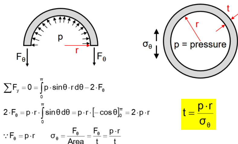
Figur 10-3. Tangentialspänning och vägg tjocklek för cylinder
