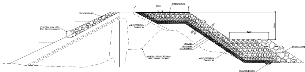
Figur 1-2. Principskiss som visar förstärkningen av Löjefors späddamm.
